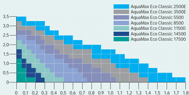
Filter- und Bachlaufpumpe AquaMax Eco Classic
